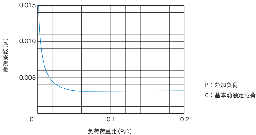
图7 负荷重比与摩擦系数的关系
